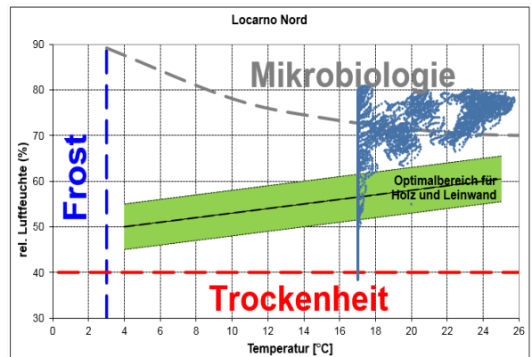
Raumklima Auswertung in einer Kirche
