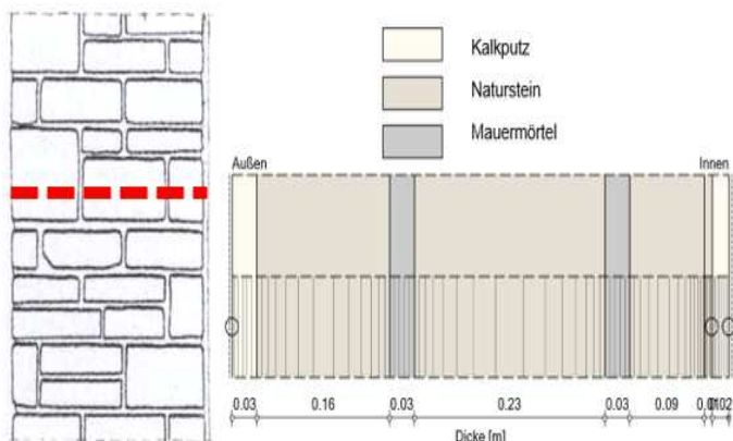
Simulation der Wärme- und Feuchteprozesse eines historischen Wandaufbaus
