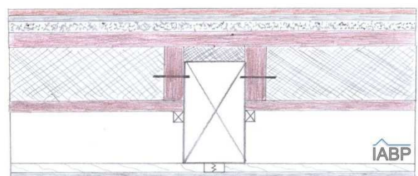
Verbesserung des Schallschutzes einer bestehenden Decke
