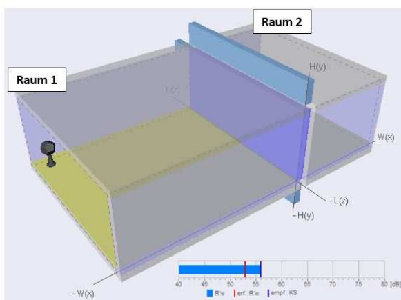
Simulation des Schallschutzes eines einschaligen Trennbauteils
