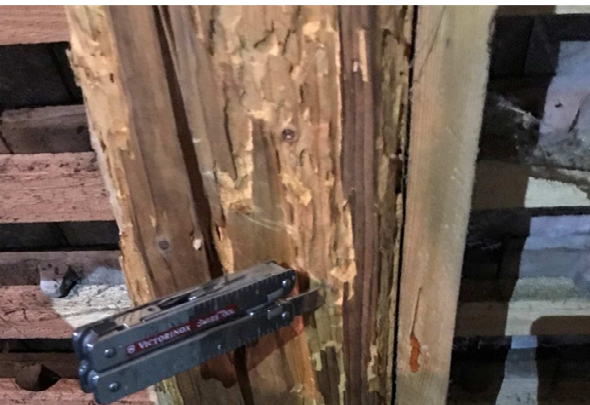
Begutachtung von Insektenbefall an Dachgebälk
